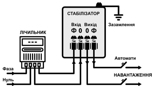
Рис.9 – Схема підключення стабілізатора до однофазної мережі
